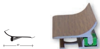
ART. 2706 - Copriangolo per gradino Lung: m 2.70. Giunzione tra l'alzata e la pedata del gradino.
