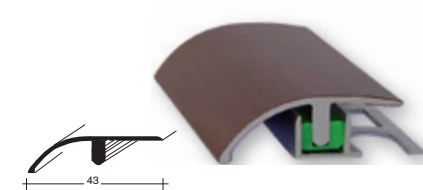
ART. 2716 - Profilo di dislivello per 12 mm. Lung: m 2.70. Per collegare due livelli di pavimento.
