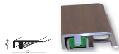
ART. 2714 - Profilo terminale Lung: m 2.70. Serve come terminale nel punto in cui si interrompe il pavimento.
