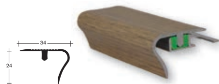
ART. 2717 - Profilo paragradino universale Lung: m 2.70. Giunzione tra pedata e alzata del gradino.
